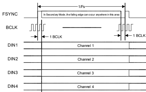
Figure 4-26. TDM Data Format—4 x DIN
