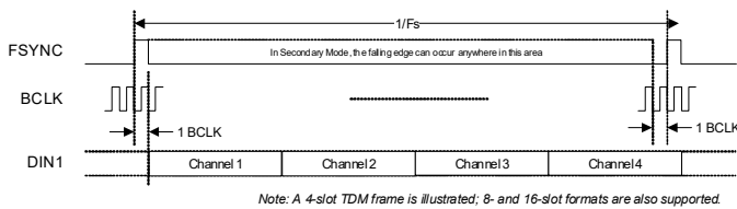
Figure 4-24. TDM Data Format—1 x DIN
