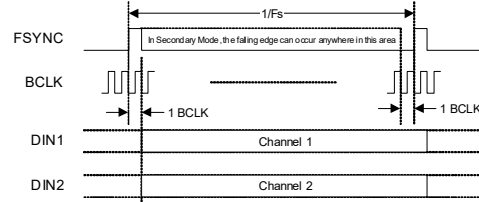
Figure 4-30. TDM Data Format—2 x DIN
