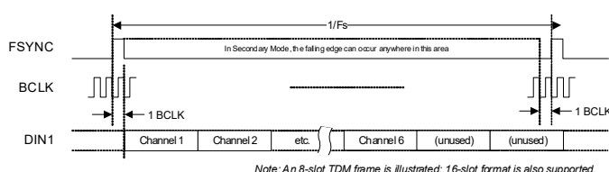
Figure 4-19. TDM Data Format—1 x DIN
