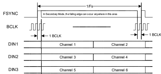
Figure 4-21. TDM Data Format—3 x DIN
