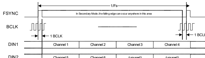
Figure 4-20. TDM Data Format—2 x DIN
