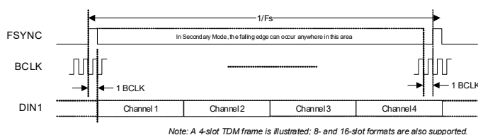
Figure 4-24. TDM Data Format—1 x DIN
