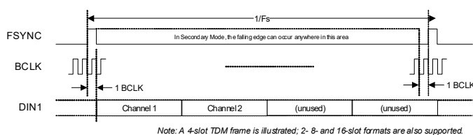
Figure 4-29. TDM Data Format—1 x DIN
