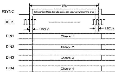
Figure 4-26. TDM Data Format—4 x DIN
