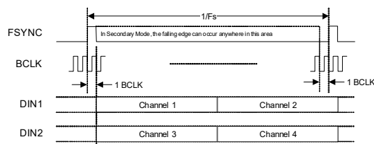
Figure 4-25. TDM Data Format—2 x DIN
