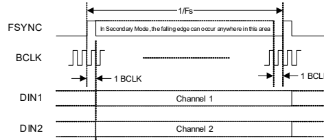
Figure 4-30. TDM Data Format—2 x DIN
